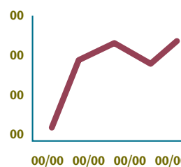
SEDIAM VENIAM NULA
